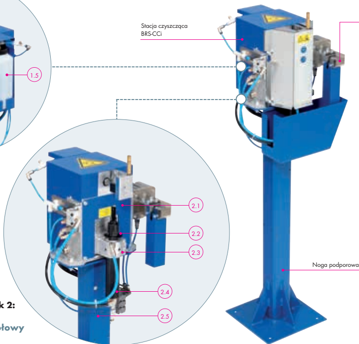
Rysunek 1: Widok tylnej części BRS-CCi
